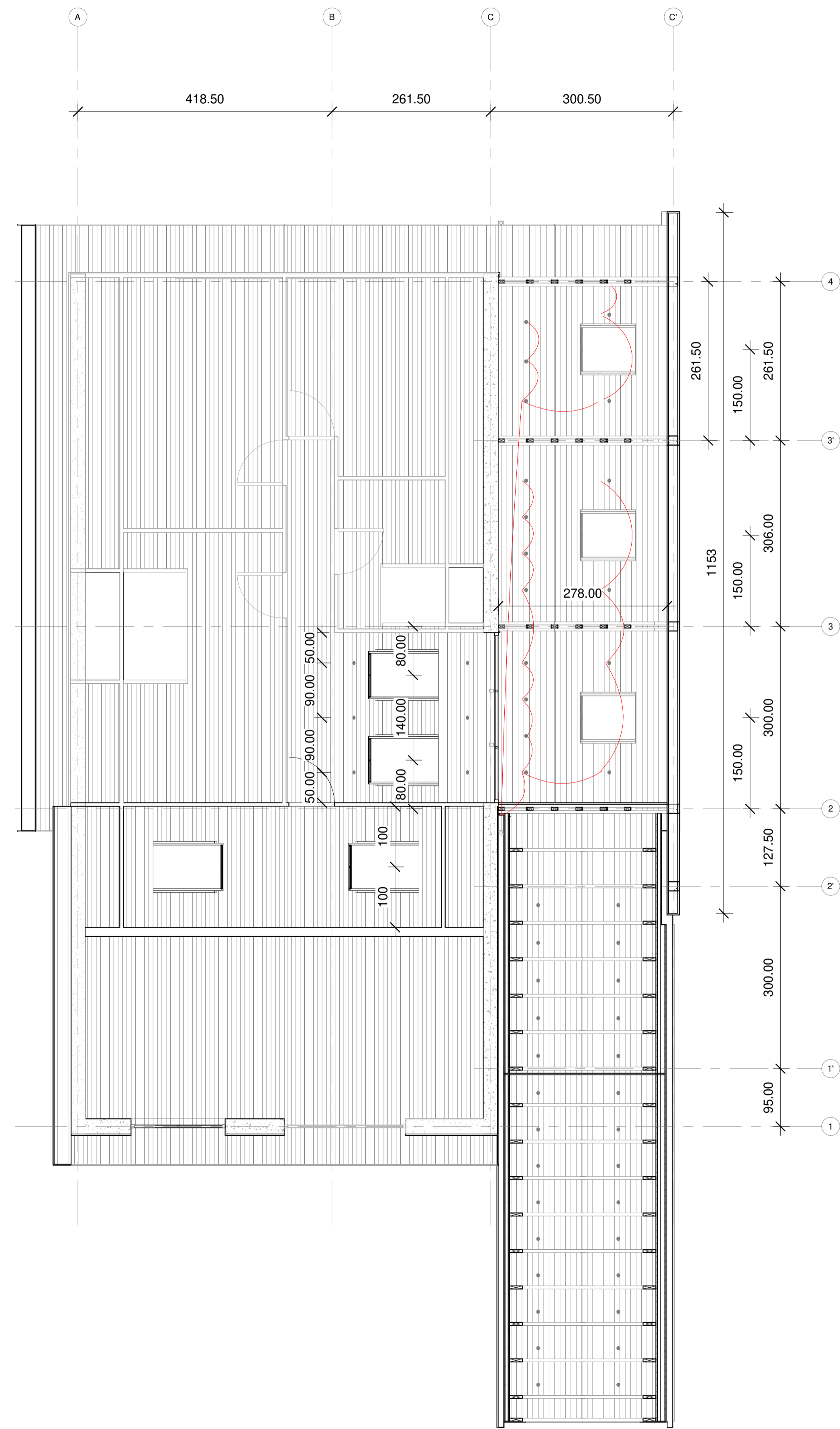
Planta Cielo Nivel 2 1 : 50
