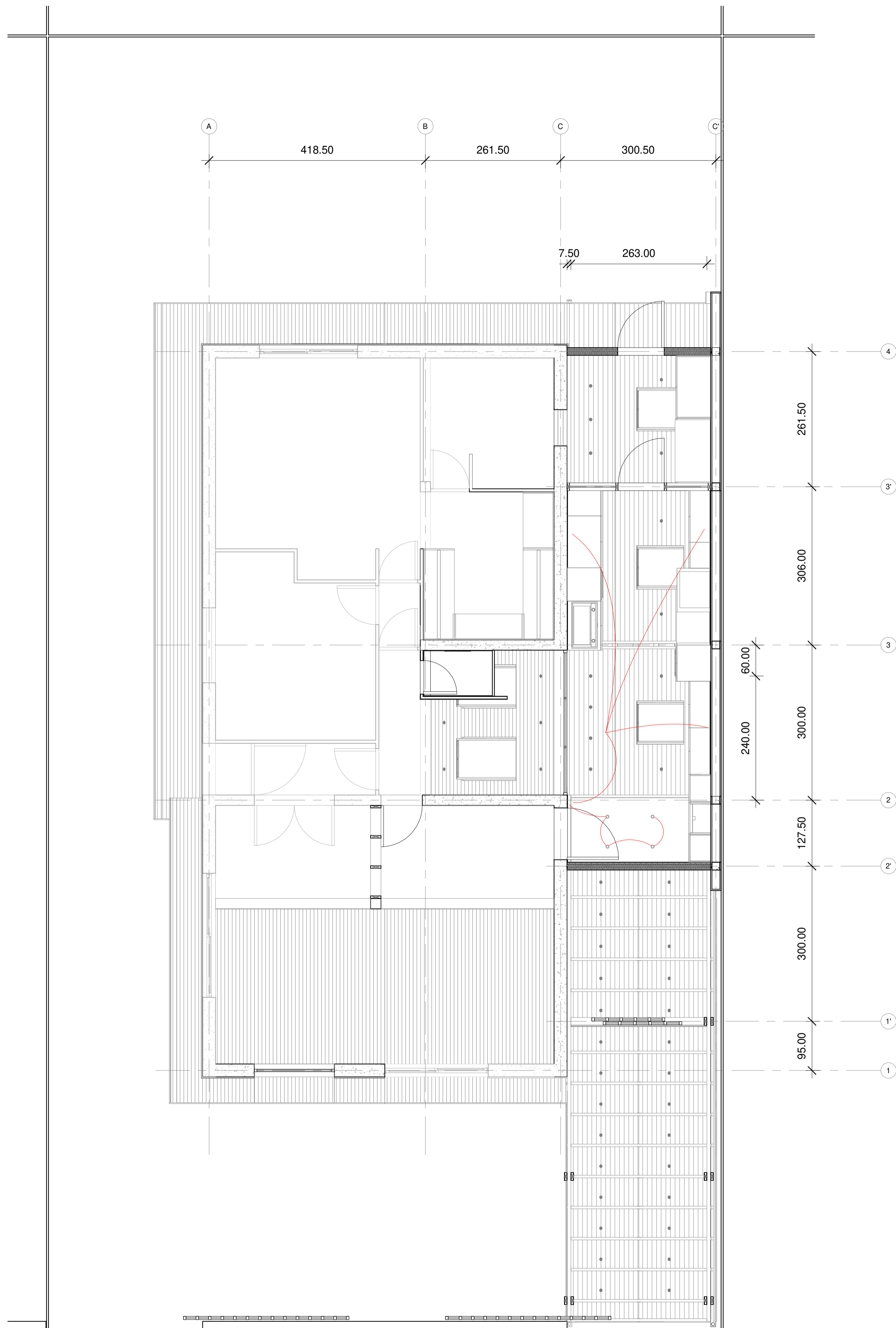
Planta Cielo Nivel 1 1 : 50
